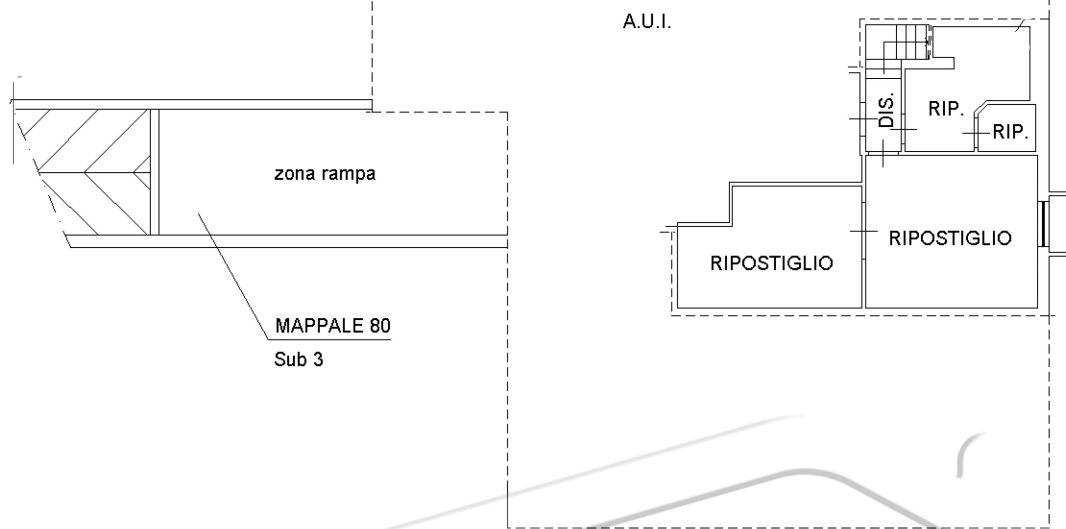
PIANTA PIANO INTERRATO
